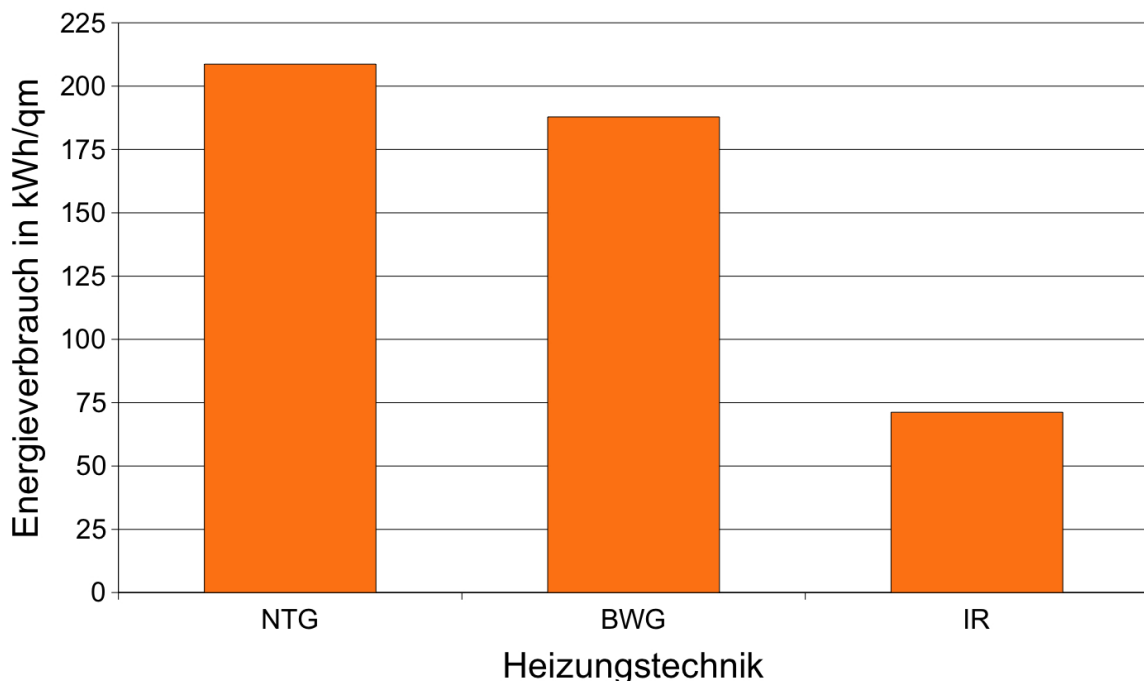
Bild 4.8: Wohnflächenbezogener Energieverbrauch im Vergleich
